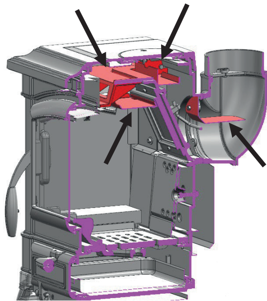
2 - RAUCHGASABWEISER
