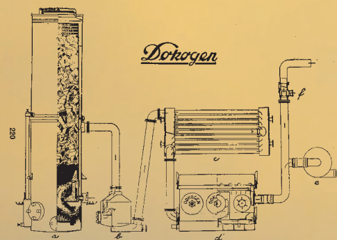
Holzvergassergenerator DOKOGEN – 1938
